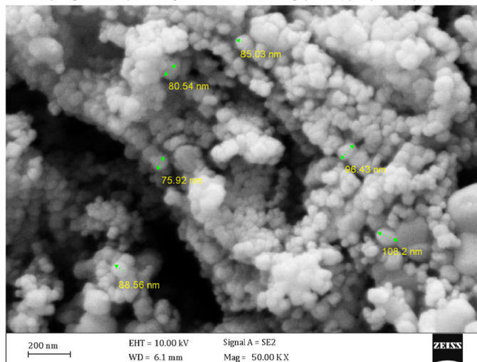
شکل ۴- تصویر میکروسکوپ الکترونی FE-SEM در مقیاس ۲۰۰ نانومتر از سطح نانوذرات سلنیم
